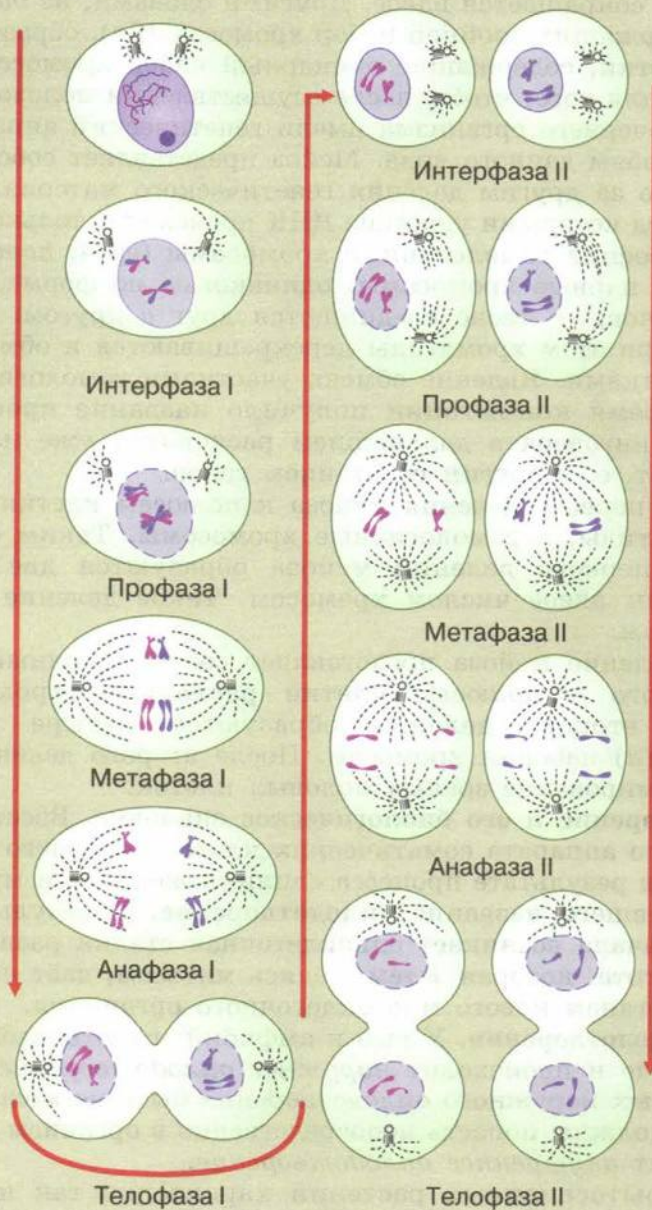
Рис. 20. Схема мейоза
